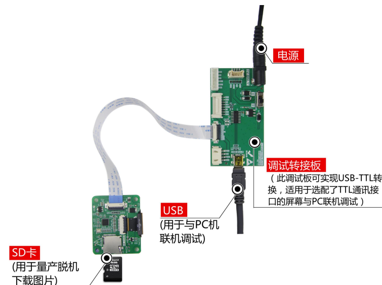
图 1-3 调试工具图
